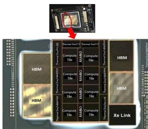
Рис. 15. Расположение чиплетов выделенной зоны процессора Ponte Vecchio [21]
